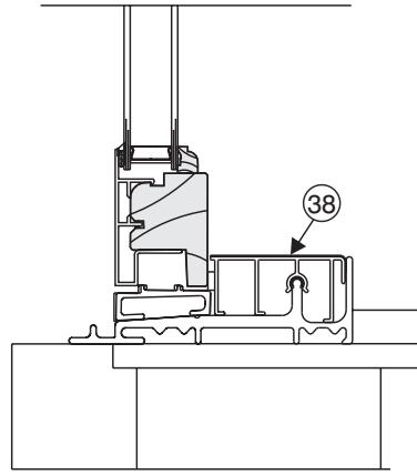
Contempra Aluma Insert w/Aluma TFT
